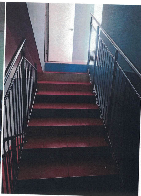
лестничный марш
